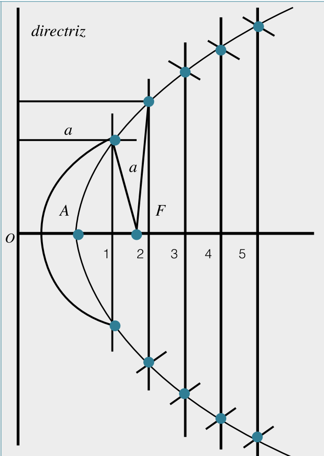
Trazo de parábola
