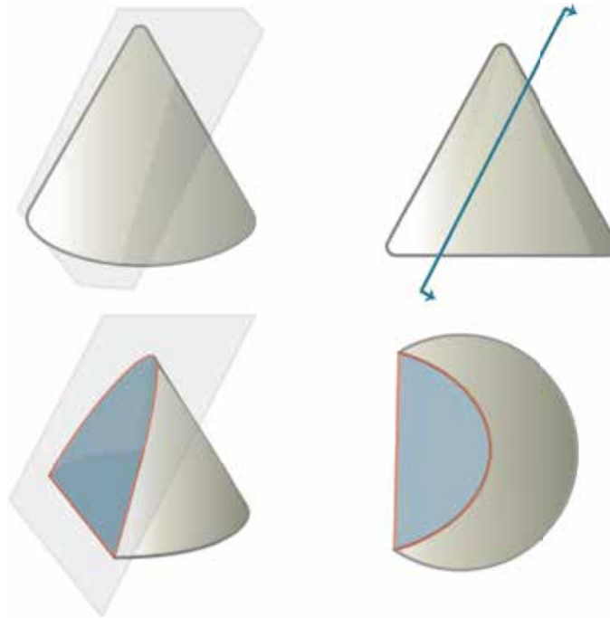
Corte a cono
