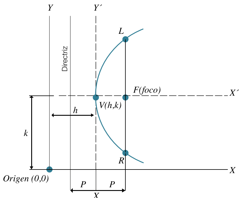
Representación gráfica de una parábola fuera del origen
